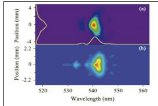
Fig. 4.3 - Tipica misura dello spettro FEL in regime di Singola Spike (a) e confronto con le simulazioni (b).
