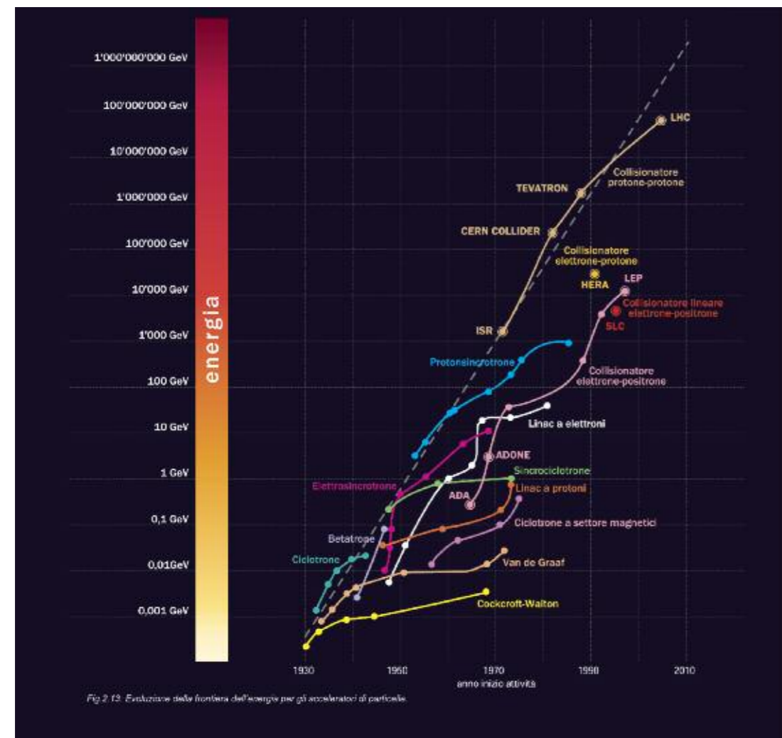
Fig. 2.13: Evoluzione della frontiera dell'energia per gli acceleratori di particelle di particelle
