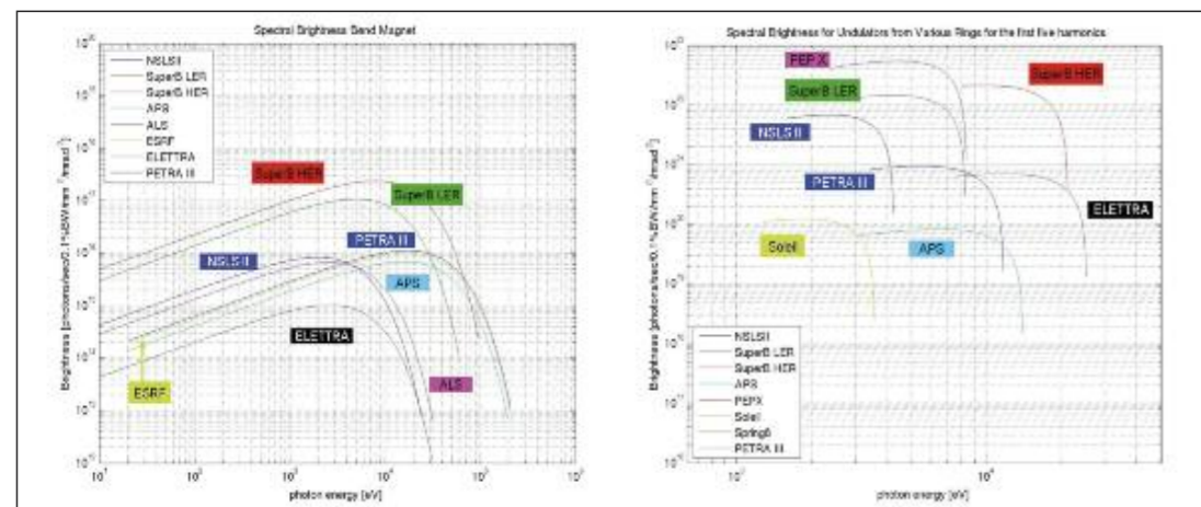
Fig. 4.26 a e b: Caratteristiche spettrali della luce di sincrotrone prodotta in SuperB nei magneti di piegatura e negli ondulatori.
