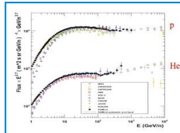
Fig. 3.8: Spettro del flusso di protoni e nuclei di elio cosmici, registrato dall'esperimento satellitare PAMELA - in orbita dal Giugno 2006.
