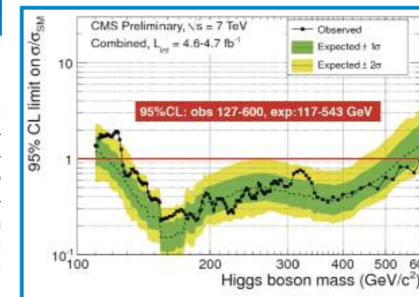
Fig. 3.2: Risultati dell'esperimento CMS sulla ricerca del bosone di Higgs. In funzione della massa del bosone di Higgs viene mostrato il limite al 95% di livello di confidenza sulla sezione d'urto di produzione normalizzata alla sezione d'urto attesa dal Modello Standard; valori inferiori a 1 escludono l'esistenza del bosone di Higgs a quella massa con questo livello di confidenza (CERN, 13 dicembre, 2011).
