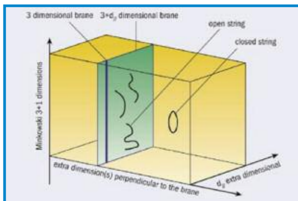
Fig. 3.14 Rappresentazione schematica di un "brane-world", con stringhe (aperte o chiuse) e dimensioni extra (da un disegno del Cern Courier).
