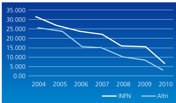
Fig. 11.3: Media delle citazioni fino a fine 2010 per articoli pubblicati negli anni 2004-2010 su Physical Review D (sinistra) e Nuclear Physics B (destra). Le pubblicazioni INFN sono in bianco, le globali in azzurro
