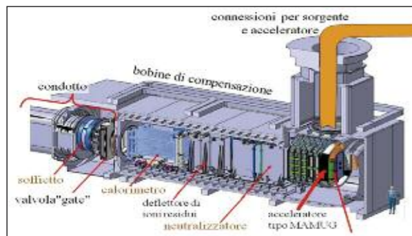
Fig. 4.16: La nuova sorgente ECR.
