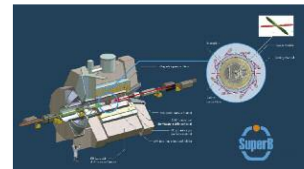
Fig. 4.27: Schema del collisore elettrone-positrone Super-B.
