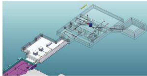
Fig. 3.22: Isometrico laboratorio Ciclotrone e layout di trasferimento e selezione del fascio esotico.
