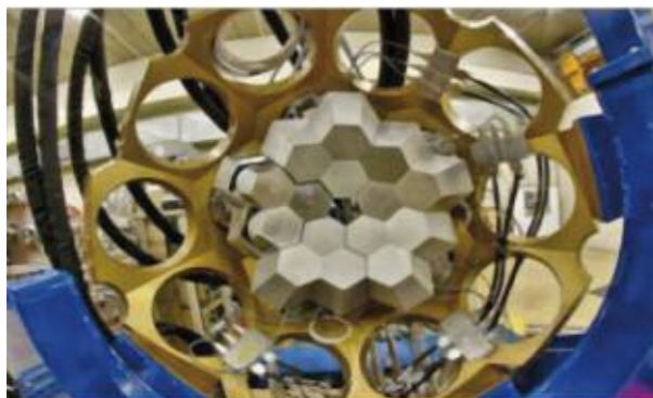
Fig. 3.13: Il dimostratore del rivelatore AGATA, che usa la tecnica del tracciamento dell'interazione gamma con la materia, montato ai Laboratori Nazionali di Legnaro.
