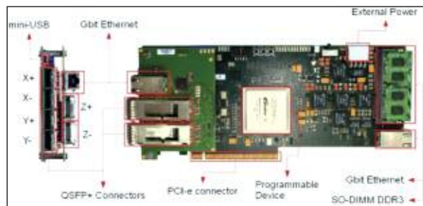
Fig. 3.19: Scheda apeNEXT+
