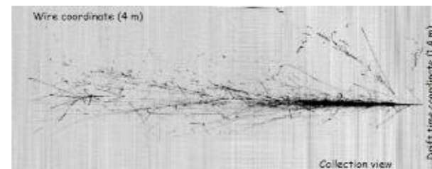
Fig. 3.7: Interazione di un \nu_\mu del CNGS osservata dal rivelatore ICARUS al LNGS
