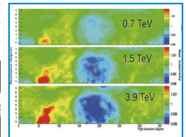
Fig. 3.10: Anisotropia nei raggi cosmici a energie dell'ordine del TeV, osservata dall'esperimento ARGO, in Tibet.
