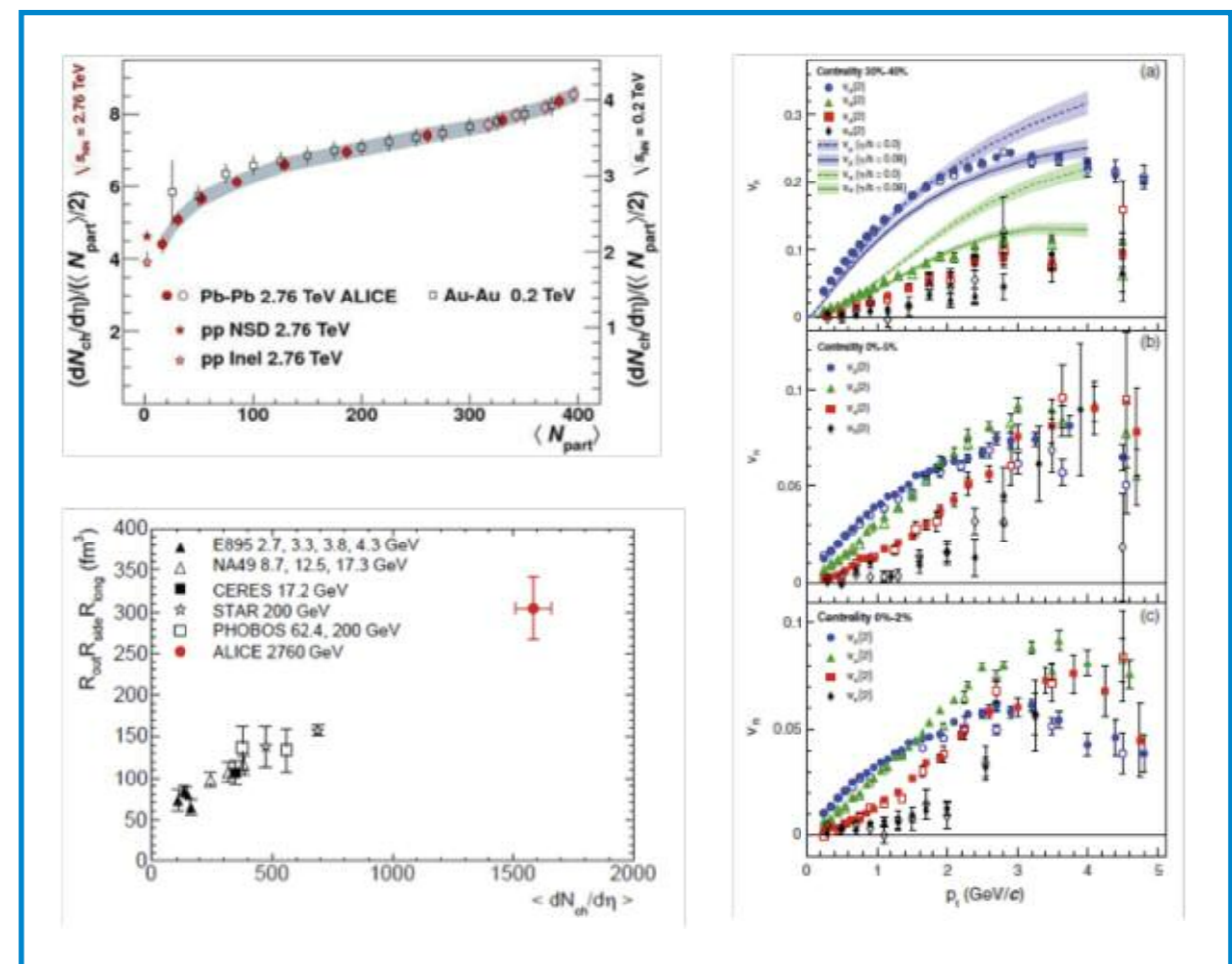
Fig. 3.12: Alcuni tra i risultati più interessanti ottenuti da ALICE nel 2011 in interazioni centrali Pb-Pb a 2.76 TeV/nucleone. A sinistra (in alto) è mostrata la densità di particelle cariche in funzione della centralità (Phys. Rev. Lett. 106, 032301 (2011)); il grafico di sinistra (in basso) mostra i risultati dell'analisi delle correlazioni HBT: prodotto R_{out} \cdot R_{side} \cdot R_{long} per kT=0.3 GeV/c (Phys. Lett. B 696 (2011) 328); In entrambi i grafici i risultati di ALICE sono paragonati con misure a energie inferiori. A destra sono mostrate le misure del flusso di particelle cariche in termini di v_2 , v_3 , v_4 , e v_5 in funzione del momento trasverso per tre differenti intervalli di centralità.
