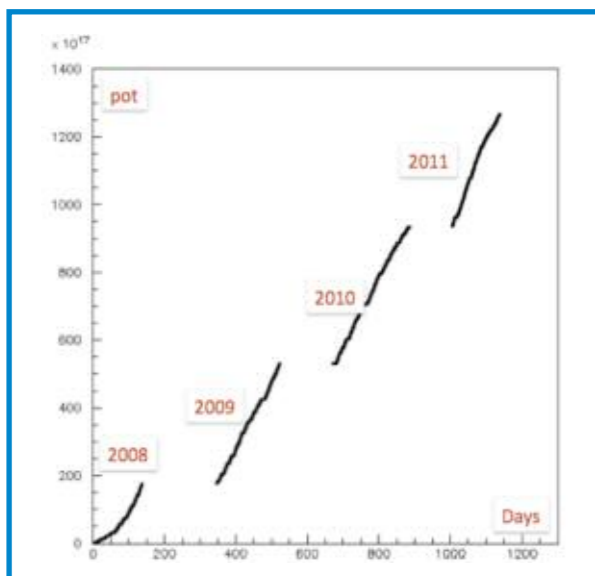
Fig. 3.6: Crescita del valore di luminosità integrata di CNGS dal 2008 al 2011.
