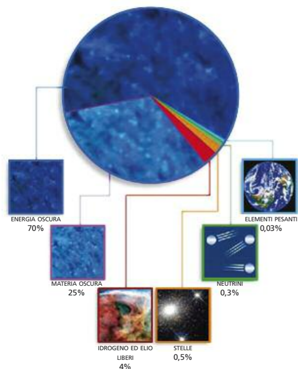
Fig.2.3: La composizione dell'Universo
